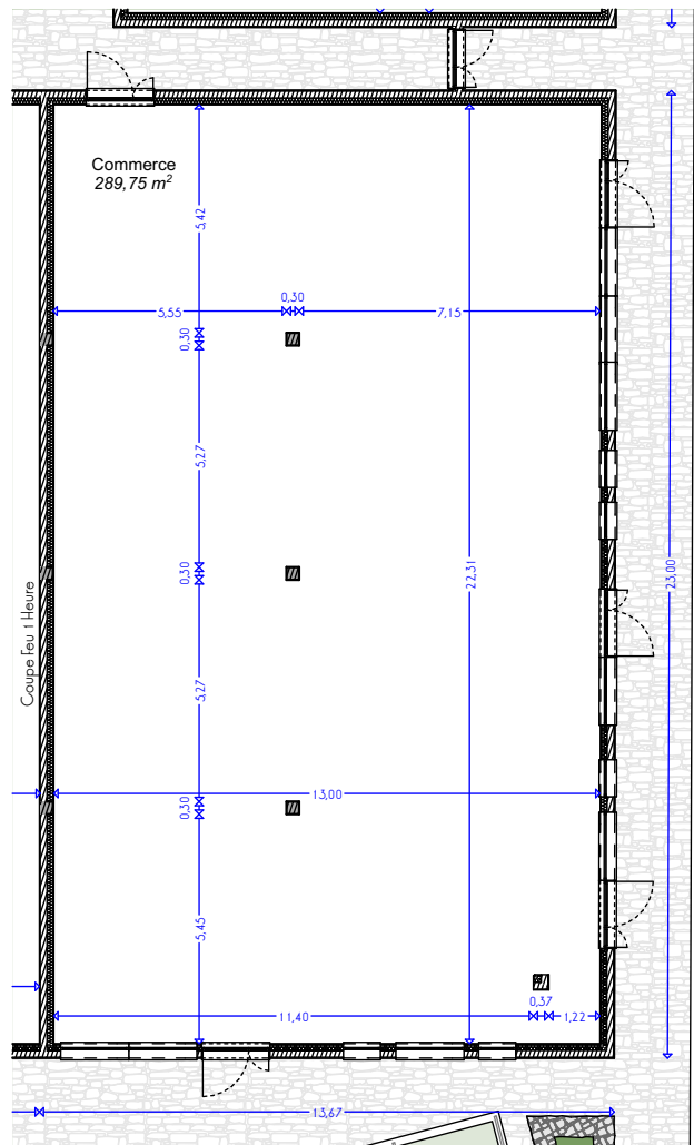
Plan du Rez - de - Jardin
